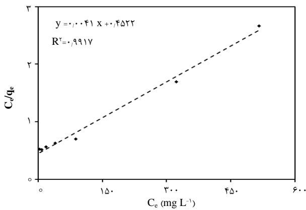
شکل ۸. نمودار خطی هم‌دمای لانگمویر برای جذب یون‌های اوراتیل بر روی SBA-۱۵-TWMP.
