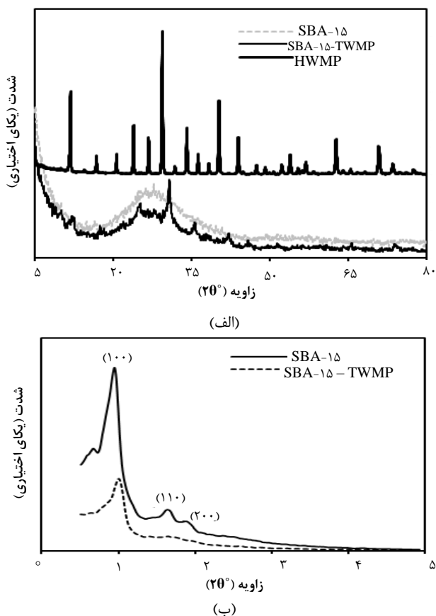
شکل ۵. الگوی پراش پرتو ایکس در SBA-15 -TWMP و SBA-15 در زاویه‌های بزرگ (الف) و کوچک (ب).
