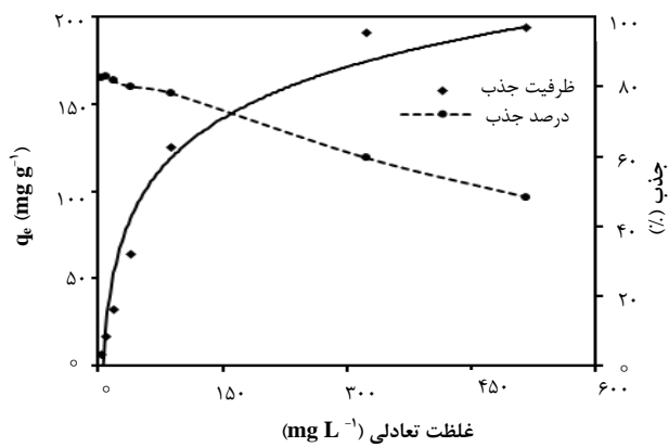
شکل ۷. همدمای جذب اورانیم بر روی SBA-15-TWMP [تندی هم‌زنی: ۱۸۰ rpm، دما: ۲۵ °C، زمان: ۲۴h، pH ۵].
