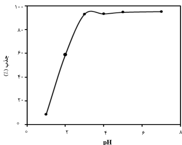
شکل ۱۱. رابطه‌ی بین pH محلول و درصد جذب یون‌های اورانیل بر روی SBA-۱۵-TWMP.
