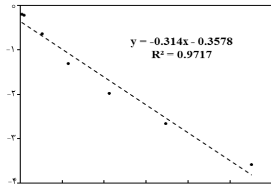
شکل ۱۰. نمودار خطی دوبینین- رادشکوچ برای جذب یون‌های اورانیل بر روی SBA-۱۵-TWMP.
