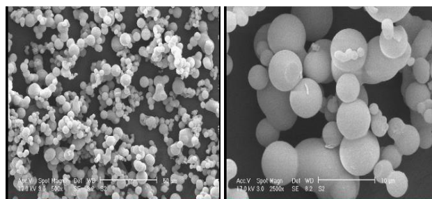
شکل ۱. تصویرهای SEM ترکیب SBA-۱۵.
