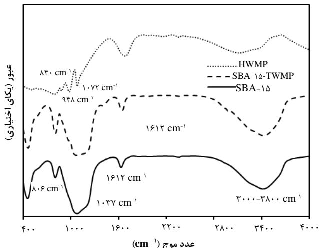
شکل ۴. طیف تبدیل فوری‌ی زیرقرمز SBA-15 ، HWMP و SBA-15 -TWMP [۳۸].
