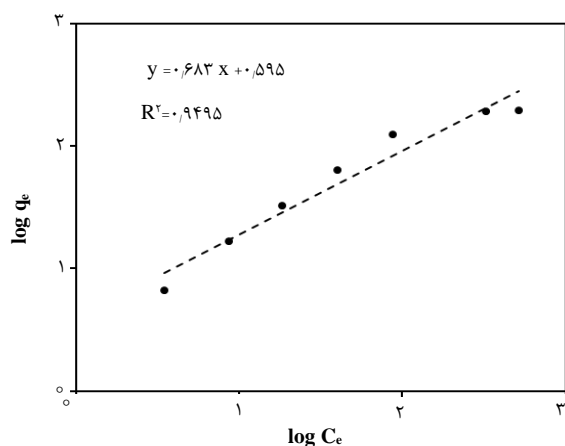
شکل ۹. نمودار خطی هم‌دمای فروندلیچ برای جذب یون‌های اوراتیل بر روی SBA-۱۵-TWMP.
