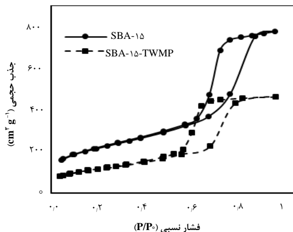
شکل ۲. هم‌دمای جذب و واجذب نیتروژن برای SBA-۱۵ و SBA-۱۵-TWMP.
