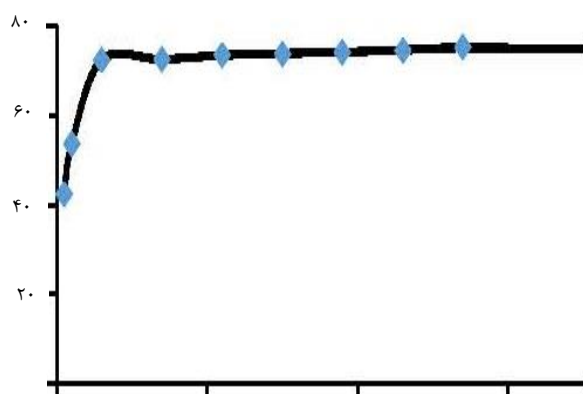
شکل ۶. تأثیر pH بر میزان حذف سرب توسط جاذب MG/ZnO. [زمان ماند ۱۰ دقیقه، تندی هم‌زنی ۲۵۰ دور در دقیقه، مقدار جاذب 0.3 \text{ g L}^{-1} ].
