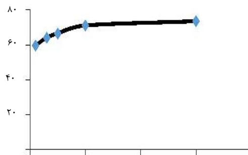
شکل ۵. تأثیر مقدار جاذب MG/ZnO بر میزان حذف سرب.
