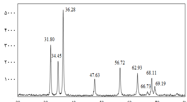
شکل ۲. الگوی پراش پرتو ایکس نانوذرات روی اکسید.
