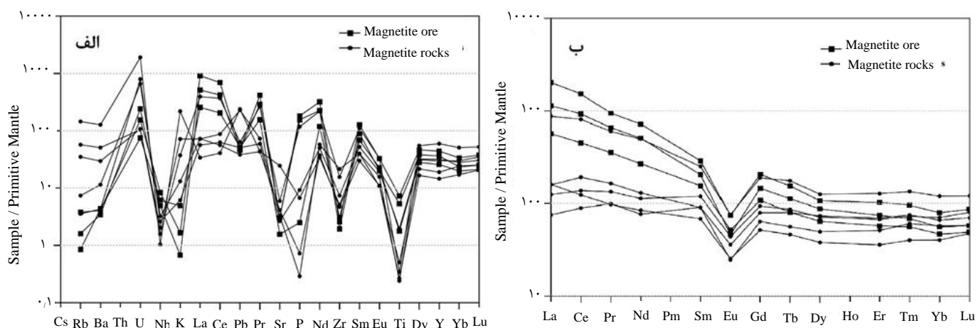
شکل ۴. نمودارهای عنکبوتی عناصر کمیاب و خاکی نادر بهنجار شده نسبت به الف) جبهه‌ی اولیه [۱۴] و ب) کندریت [۱۵] برای تعدادی از نمونه‌های حوزه‌ی برشی و کان‌سنگ مگنتیت در کانسار سه‌چاهون.
