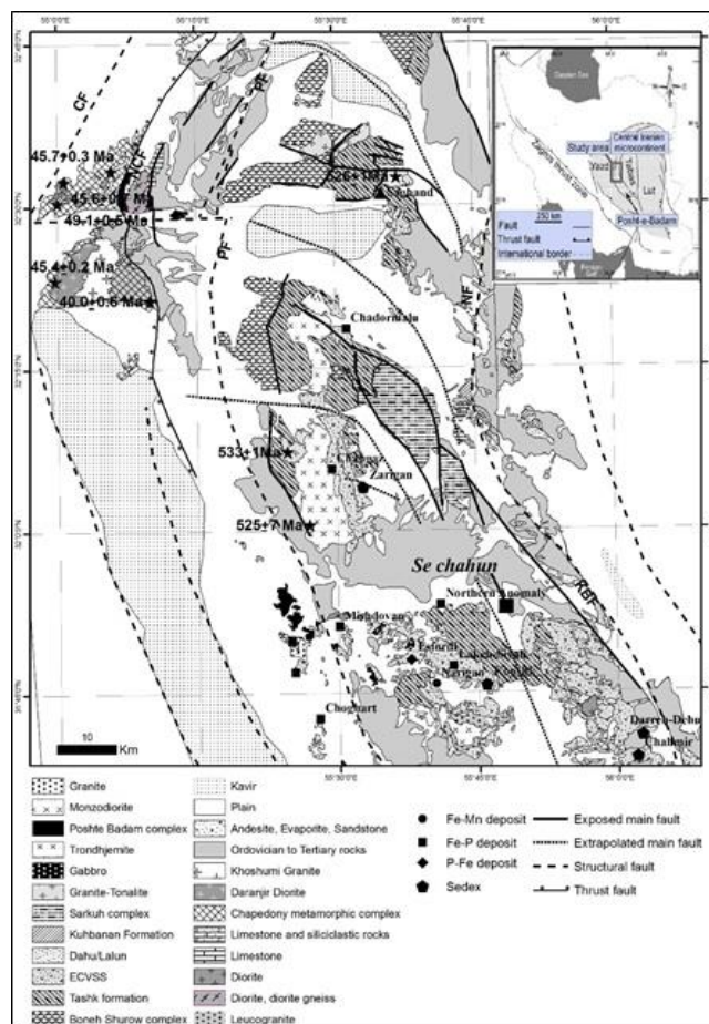
شکل ۱. نقشه‌ی زمین‌شناسی ساده شده‌ی منطقه‌ی بافق [۶، ۷، ۱۳].
