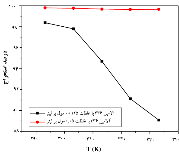
شکل ۷. اثر تغییرات دما بر درصد استخراج اورانیم. [غلظت اورانیم، 750 \text{ mg L}^{-1} ؛ غلظت سولفوریک اسید، 0.015 \text{ mol L}^{-1} ؛ نسبت فاز، ۱؛ زمان تماس، ۳۰ min]
