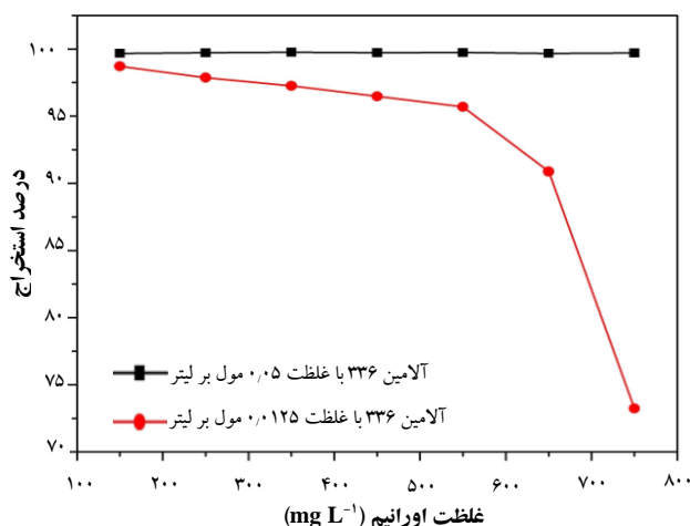
شکل ۵. اثر غلظت اورانیم محلول خوراک بر درصد استخراج اورانیم. [غلظت سولفوریک اسید، 0.015 \text{ mol L}^{-1} ؛ نسبت فاز، ۱؛ دما: 25^\circ \text{C} ؛ زمان تماس، ۳۰ min]
