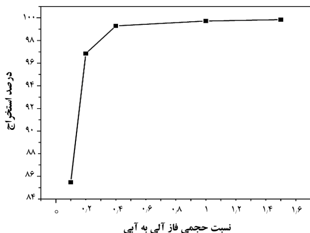
شکل ۶. اثر نسبت فاز آلی به آبی بر درصد استخراج اورانیم. [غلظت اورانیم، 750 \text{ mg L}^{-1} ؛ غلظت سولفوریک اسید، 0.015 \text{ mol L}^{-1} ؛ غلظت آمونیاک، 0.005 \text{ mol L}^{-1} ؛ دما، 25^\circ \text{C} ؛ زمان تماس، ۳۰ min]
