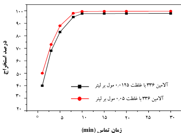
شکل ۲. اثر زمان تماس بین فازها بر درصد استخراج اورانیم. [غلظت اورانیم، 250 \text{ mg L}^{-1} ؛ نسبت فاز، ۱؛ دما: 25^\circ\text{C} ؛ غلظت سولفوریک اسید، 0.15 \text{ mol L}^{-1} ]
