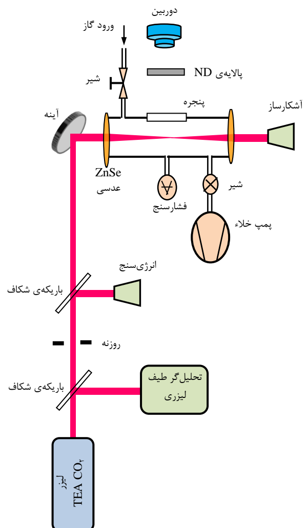
شکل ۱. ترتیب آزمایشی انجام استفاده شده.
