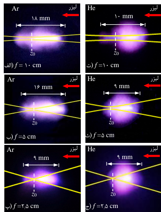
شکل ۶. تصویر جرقه‌های لیزر- القا در فشار ۴۰۰ mbar در گازهای آرگون (چپ) و هلیم (راست) برای فاصله‌های کانونی گوناگون، همراه با مسیر پرتوهای لیزری مربوطه.
