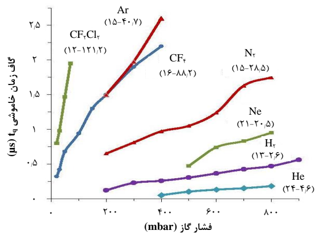
شکل ۵. تغییرات پهنای گاف زمان خاموشی با فشار برای گازهای گوناگون و با فاصله‌ی کانونی ۲٫۵ cm. f = 2.5 cm. عددهای داخل پرانتز، وزن مولکولی و انرژی یونش ( M-\varepsilon ) گازها است.
