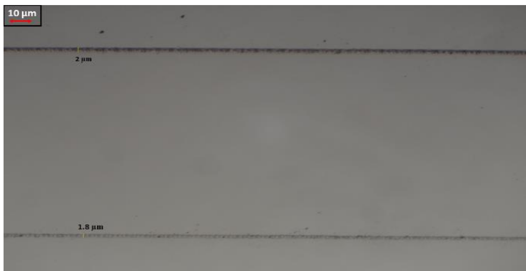
شکل ۵. ریزنگاره‌ی میکروسکوپ نوری عبوری از رد به‌جامانده در اثر برهم‌کنش تپ‌های لیزر فمتوثانیه با نمونه‌ی شیشه‌ای برای جابه‌جایی‌های نمونه با سرعت‌های مختلف: بالای تصویر، v_1 = 0.02 \text{ mm s}^{-1} و پایین تصویر، v_2 = 0.05 \text{ mm s}^{-1} .
