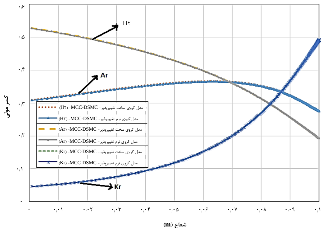
شکل ۱۲. نمودار تغییرات شعاعی غلظت گازهای درون روتور یک ماشین سانتریفوژ، به دست آمده از دو مدل برخورد کروی سخت تغییرپذیر و کروی نرم تغییرپذیر در سرعت چرخشی دیواره تا 400 \text{ m s}^{-1} .
