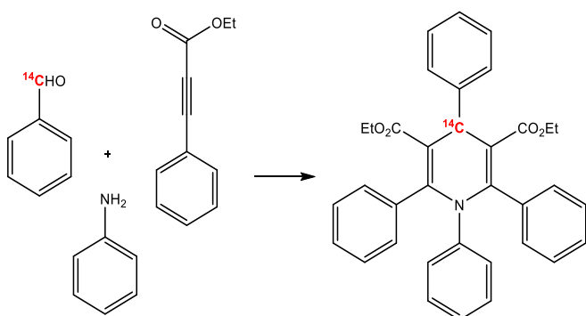
شکل ۵. طرح کلی ساخت N-فنیل-۵،۳-دی‌کربوکسیلات-۴،۱-تری‌فنیل-۴،۱-دی‌هیدروپیریدین.
