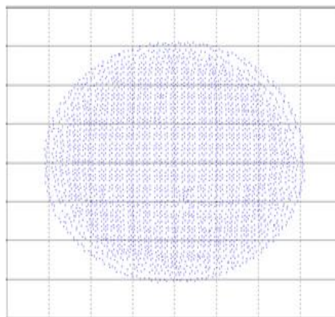
شکل ۵. نمایه‌ی ذره‌های خروجی از تفنگ الکترونی با کاتد مسطح.
