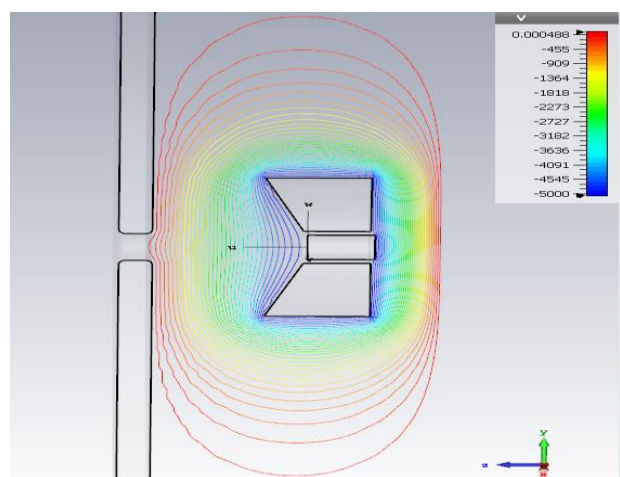
شکل ۹. خطوط میدان الکتریکی.
