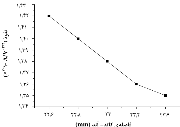
شکل ۶. رابطه‌ی بین نفوذ و فاصله‌ی کاتد-آند.
