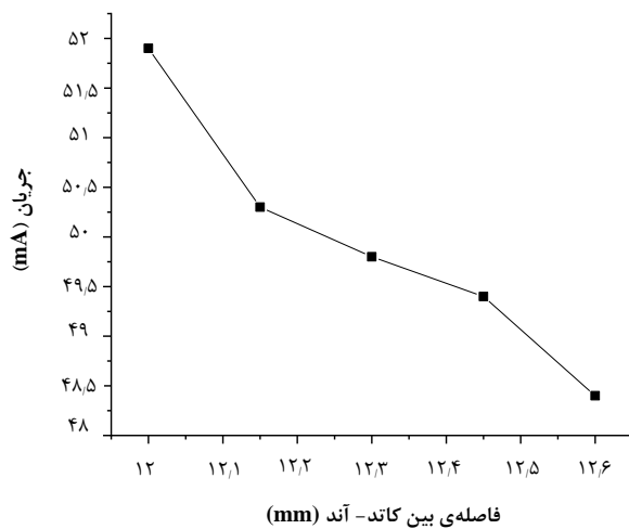
شکل ۱۶. تغییرات جریان برحسب فاصله‌ی بین کاتد و آند.
