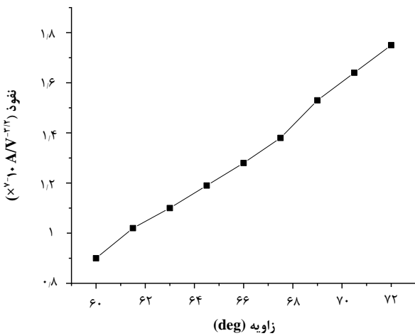
شکل ۴. رابطه‌ی بین نفوذ و زاویه‌ی الکتروود متمرکزکننده.
