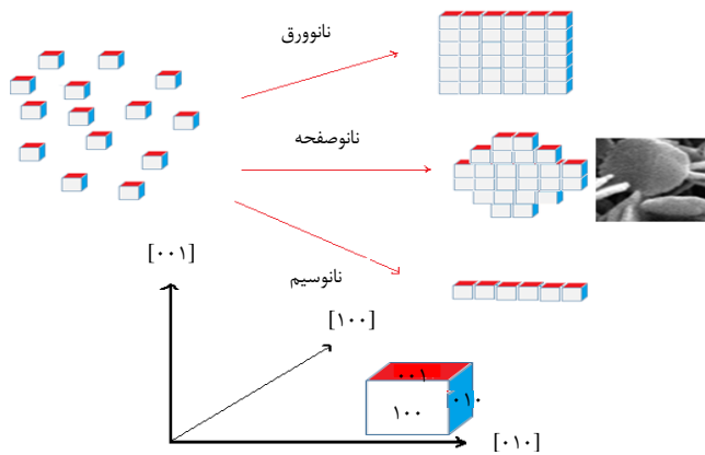
شکل ۴. طرح کلی تشکیل نانوسیم، نانوصفحه، و نانوورقها [۲۰، ۲۱].
