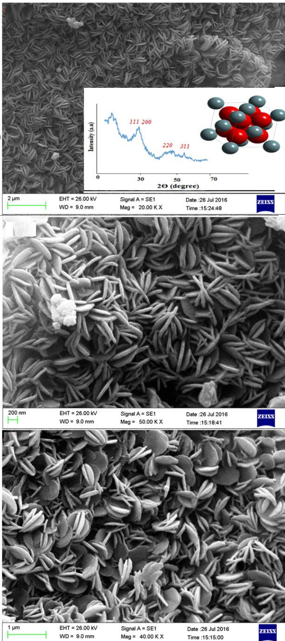
شکل ۱. ریزنگارهای میکروسکوپی الکترون پویشی (در بزرگنمایی‌های مختلف) و الگوی پراش پرتو ایکس نمونه‌ی تهیه شده در چگالی جریان 10 \text{ mA cm}^{-2} و زمان نهشت ۱۰ دقیقه.
