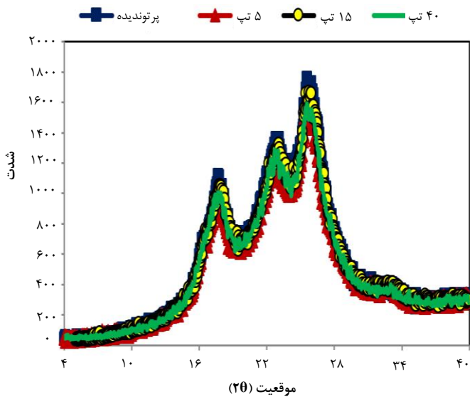
شکل ۷. الگوی پراش پرتو ایکس الیاف پلی استر.
