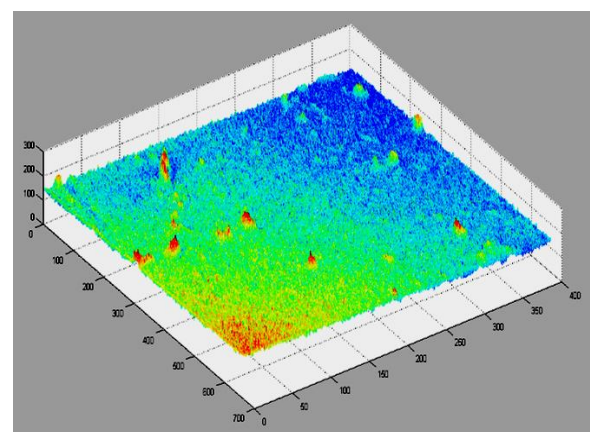
شکل ۵. تصویر سه‌بعدی سطح الیاف پلی‌استر پرتو ندیده.
