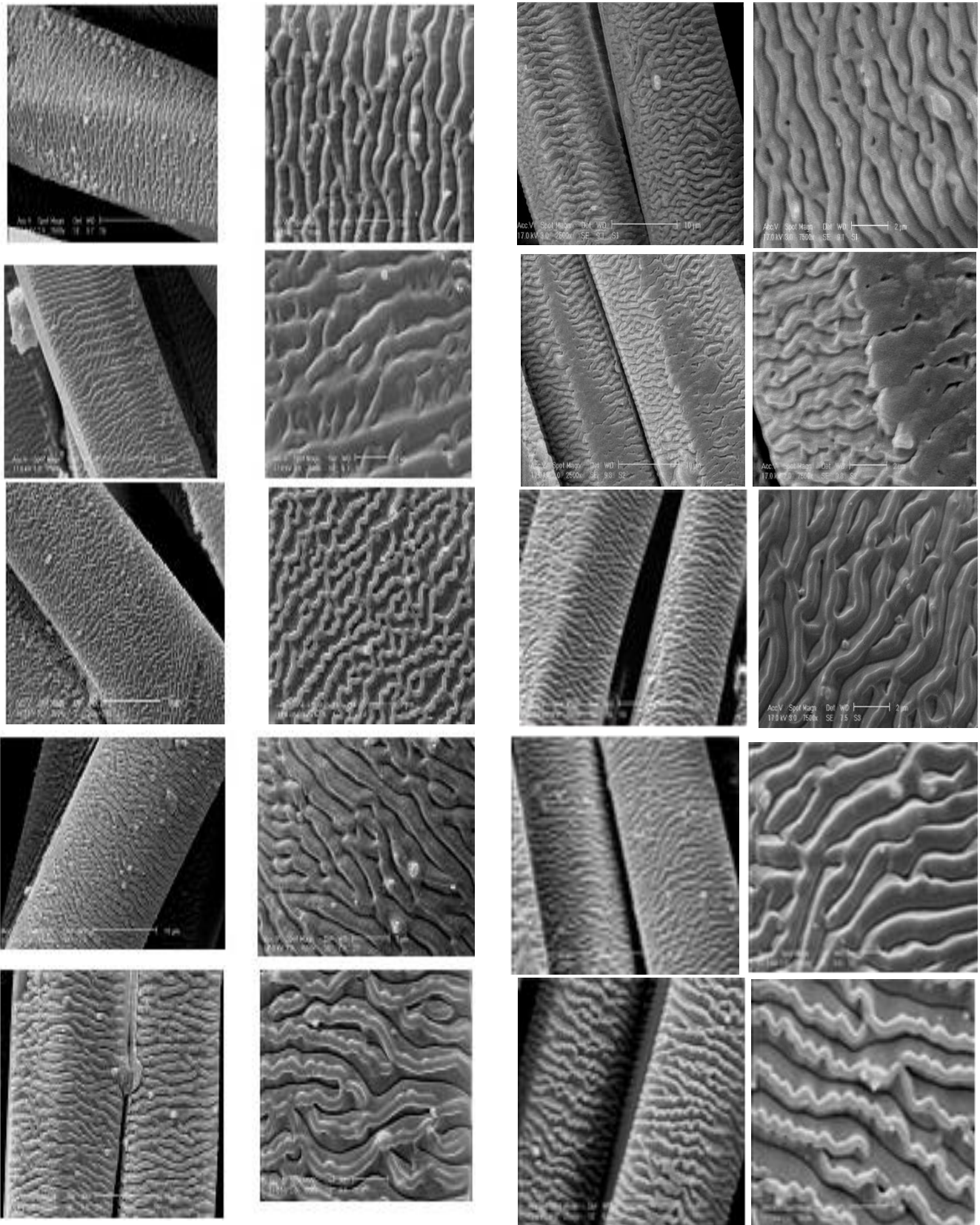
شکل ۴. تصویرهای SEM با بزرگ‌نمایی ۷۵۰۰ (سمت راست) و ۲۵۰۰ (سمت چپ) الیاف پلی استر پرتوده‌ی شده با تعداد متفاوت (به ترتیب از بالا به پایین ۵، ۱۰، ۱۵، ۲۰ و ۴۰) تپ باریکه‌ی لیزر بعد از عملیات رنگرزی.
