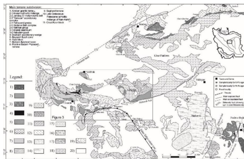
شکل ۲. نقشه‌ی زمین‌شناسی ساده‌شده‌ی منطقه‌ی انارک، جندق و پشت بادام (ایران مرکزی) [۷].
