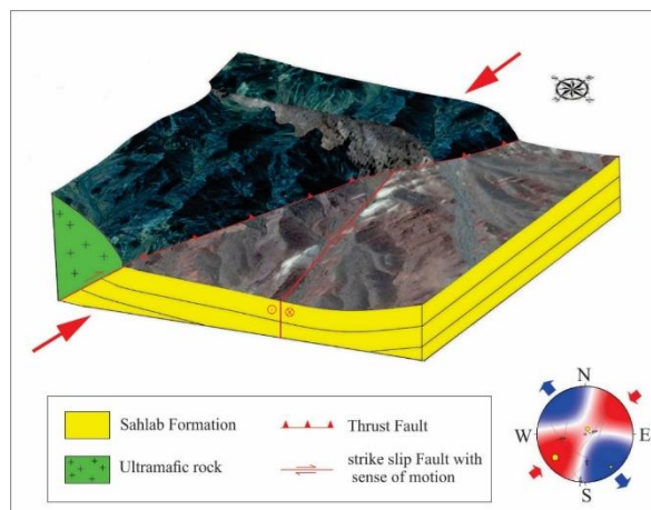
شکل ۱۲. نمایش سه‌بعدی پایان شکل‌گیری و تکامل لیستونیت‌ها بین لایه‌های اولترامافیک در پاسخ به فاز دوم تنش.
