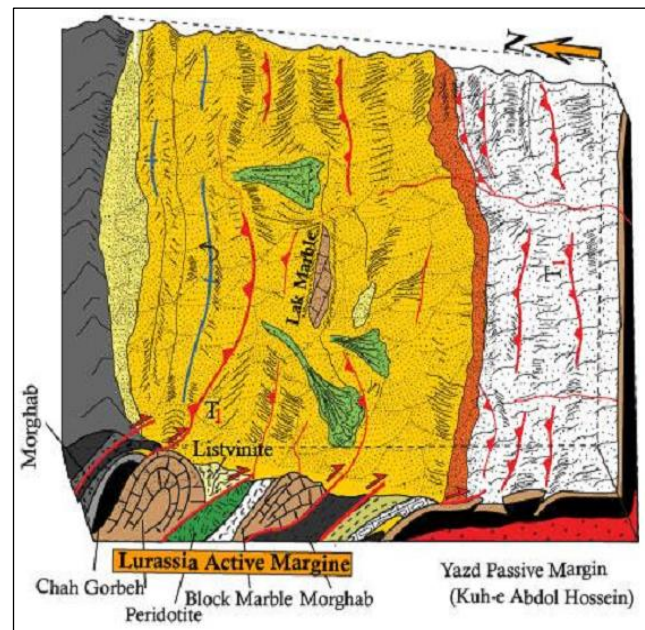
شکل ۳. مدل طرح‌وار در زمان تریاس برای موقعیت زمین‌ساختی و ارتباط واحدهای سنگی ساختاری در منطقه‌ی انارک [۹].
