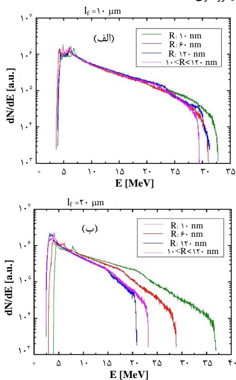
شکل ۳. طیف انرژی باریکه پروتون در هدف با لایه فومی الف) ۱۰ میکرومتری و ب) ۲۰ میکرومتری. طیف مربوط به شعاع‌های مختلف با رنگ‌های مختلف نشان داده شده است.
