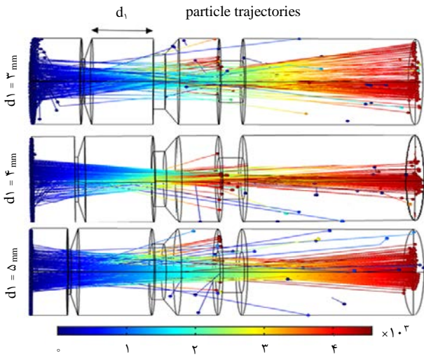
شکل ۷. تغییرات واگرایی باریکه را برحسب تغییرات فاصله بین دو الکتروود اول با در نظر گرفتن بار فضایی.
