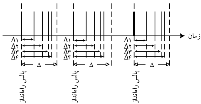
شکل ۱. الگوریتم تحلیل رُسی - آلفا نوع اول.
