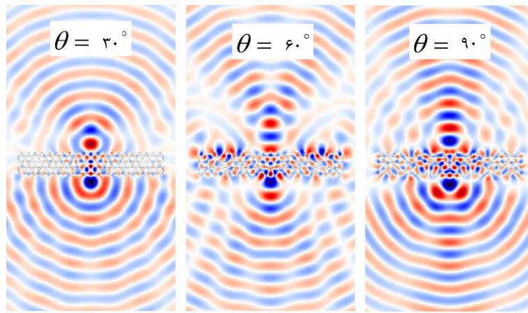
شکل ۴. توزیع میدان الکترومغناطیسی در دو سوی بلور برای حالتی که زاویه \theta تغییر کرده به ازای فرکانس فرودی (\omega = 0.3)(2\pi c/\alpha) .
