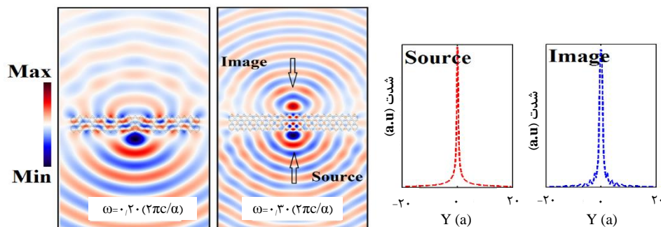
شکل ۳. تصویر ناشی از یک منبع نور با فرکانس (2\pi c/a) و 0.3(2\pi c/a) و پروفایل شدت میدان الکترومغناطیسی در محل حضور منبع و تصویر برای فرکانس (2\pi c/a) .
