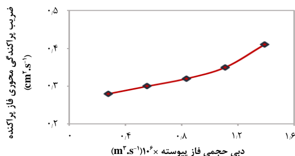
شکل ۹. اثر تغییرات دبی حجمی فاز پیوسته بر ضرایب پراکندگی محوری فازها برای استخراج اورانیم در ستون ضربه‌ای افقی (Qd=3 l/h, af=1 cm/s).
