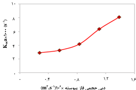
شکل ۷. اثر تغییرات دبی حجمی فاز پراکنده بر ضریب کلی حجمی انتقال جرم فاز پیوسته برای استخراج اورانیم ( af=1 cm/s, Q_c=3 l/h).
