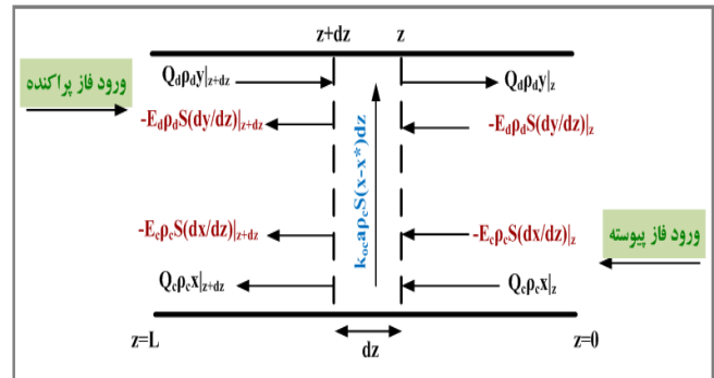
شکل ۳. المان موازنه جرمی برای مدل پراکندگی محوری.
