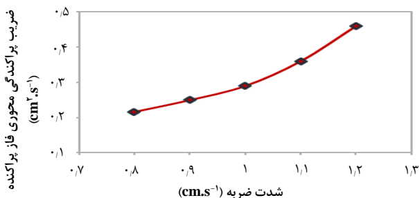
شکل ۸. اثر تغییرات شدت ضربه بر ضرایب پراکندگی محوری فازها برای استخراج اورانیم در ستون ضربه‌ای افقی (Qc=Qd=3 l/h).
