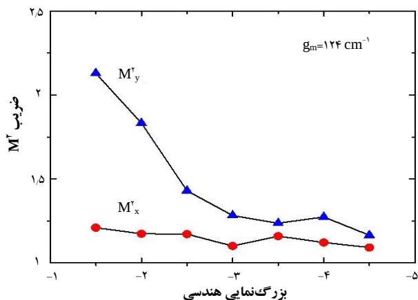
شکل ۹. رفتار ضرب کیفیت پرتو M^2 به ازای مقادیر گوناگون بزرگ‌نمایی هندسی تشدیدگر.
