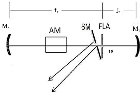
شکل ۵. آرایش تشدیدگر ناپایدار خودپالاینده: M_1 و M_2 آینه‌های چندلایه‌ای مقعر با فواصل کانونی f_1 و f_2 ؛ AM محیط تقویت کننده؛ SM آینه Scraper؛ FLA روزنه‌ی محدود کننده‌ی میدان.
