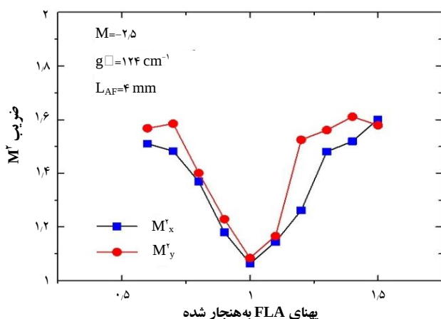
شکل ۱۱. مقادیر محاسبه شده ضریب M^r در راستای x و y به ازای مقادیر به‌هم‌نجار شده پهنای روزنه‌ی محدودکننده‌ی میدان، a_{FLA} / a .
