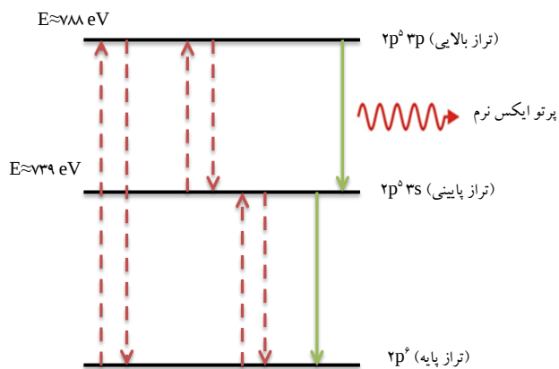
شکل ۱. ترازهای یون شبه نئون آهن Fe^{16+} برای مدل سه ترازلی لیزر پرتو ایکس ( \rightarrow گذار تابشی و \leftarrow گذار برخوردی).
