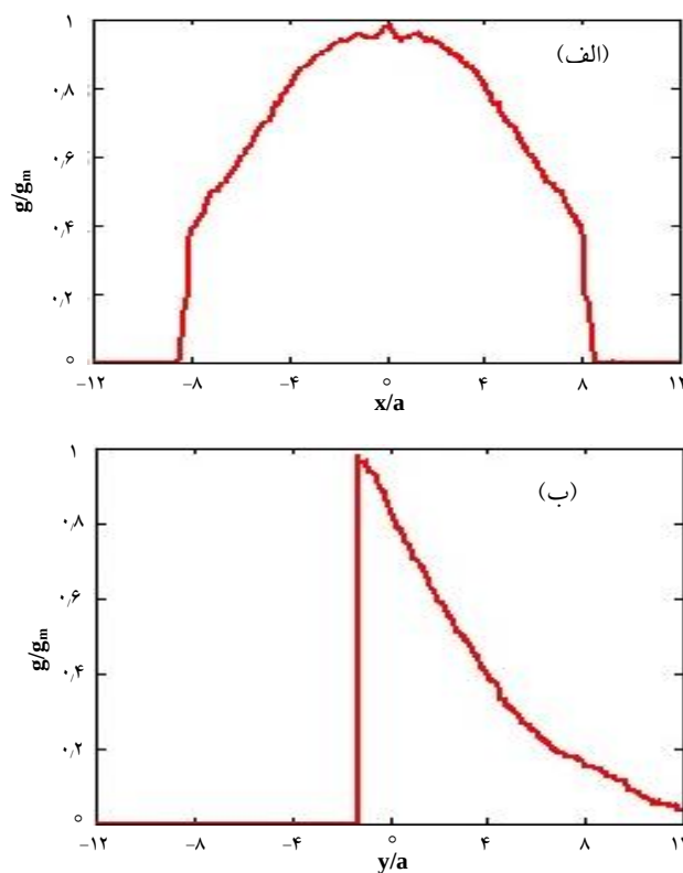
شکل ۴. ضریب بهره‌ی دو بُعدی در راستای X و Y، به‌هنگار شده نسبت به بیشینه ضریب بهره ( g_m = 124 \text{ cm}^{-1} ). مختصات نیز به شعاع روزنه، a = 7.15 \text{ } \mu\text{m} به‌هنگار شده است.
