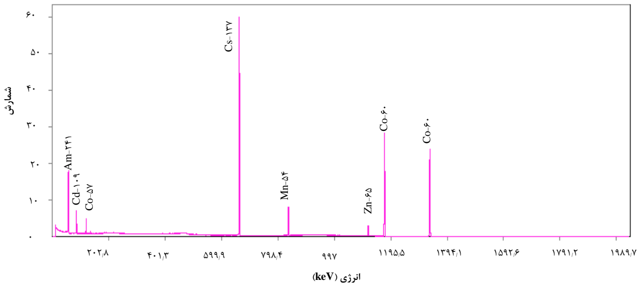
شکل ۳. طیف گامای فیلتر ساخته شده که با طیف‌سنج HPGe شمارش شده است.
