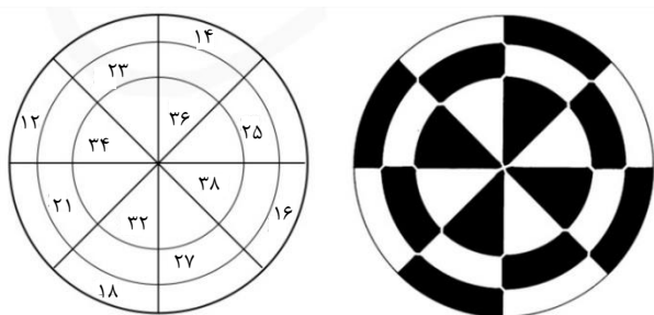
شکل ۱. نمایی از طرح پیاده شده بر روی فیلتر هپا (شکل سمت راست)، محلول استاندارد با اکتیویته معلوم بر روی قسمت‌های مشکی رنگ نشانده شده است. شماره قطعات مشکی رنگ بریده شده در شکل سمت چپ مشخص شده است.
