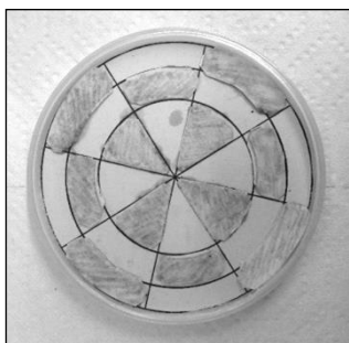
شکل ۲. نمونه فیلتر ساخته شده به عنوان چشمه استاندارد کالیبراسیون.
