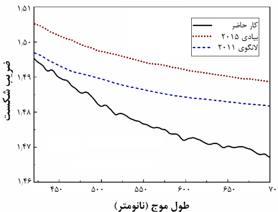
شکل ۷. تغییرات ضریب شکست در ناحیه مرئی برای الف) نمونه اولیه و نمونه‌های تابش دیده در شاریدگی‌های مختلف لیزر گاز گرنیک [۲۰] و ب) نمونه اولیه اندازه‌گیری شده در این کار در مقایسه با کار لانگوی ۲۰۱۱ [۴۲] و بیادی ۲۰۱۵ [۴۳].
