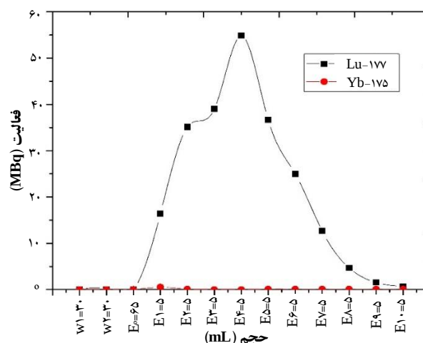
شکل ۴. کروماتوگرافی حاصل از شمارش برش‌های جمع‌آوری شده در جداسازی ^{177}\text{Lu} از هدف ایتیریم غنی شده پرتودهی شده.
