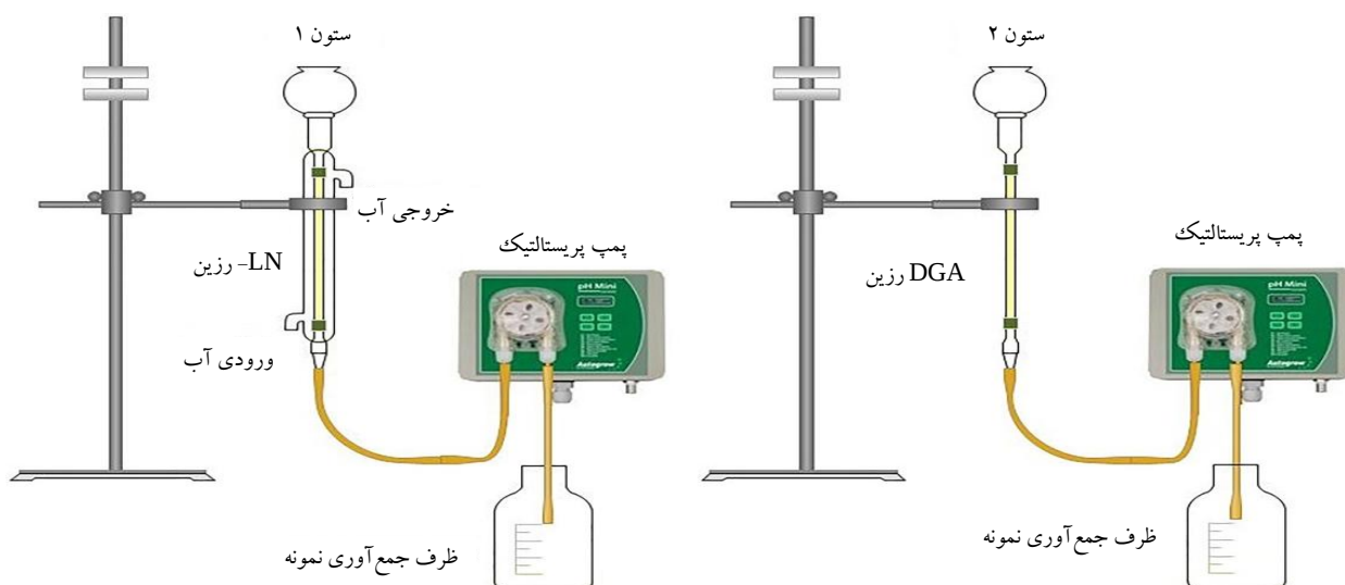
شکل ۲. سیستم‌های جداسازی تشکیل شده از ستون حاوی رزین، پمپ پرستالتیک و ولوله.
