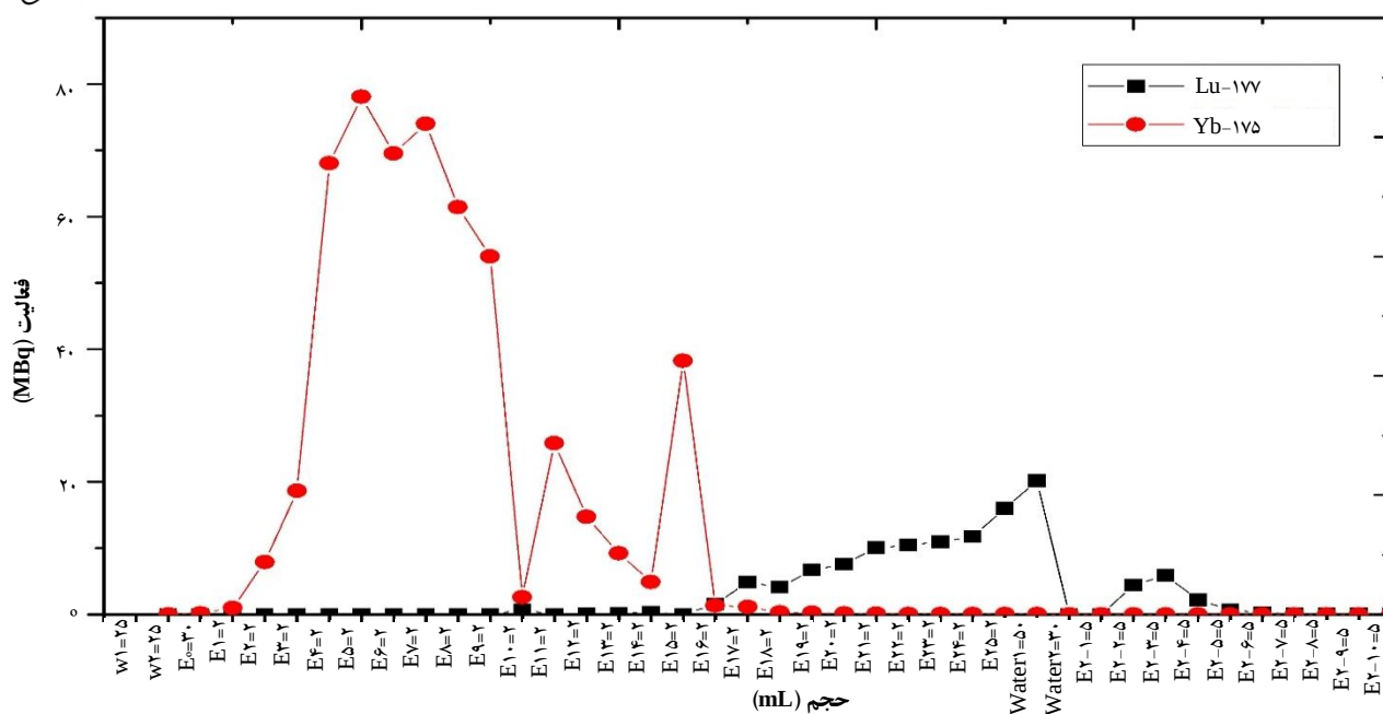
شکل ۳. کروماتوگرافی حاصل از شمارش برش‌های جمع‌آوری شده در جداسازی ^{177}\text{Lu} از هدف ایتیریم طبیعی پرتودهی شده.
