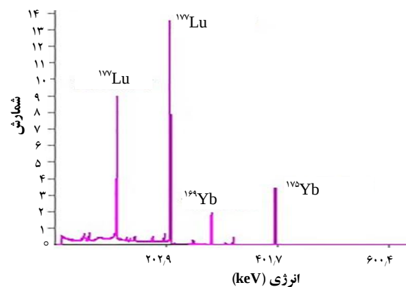
شکل ۵. طیف گامای حاصل از نمونه‌ی پرتودهی شده قبل از بارگذاری به ستون.
