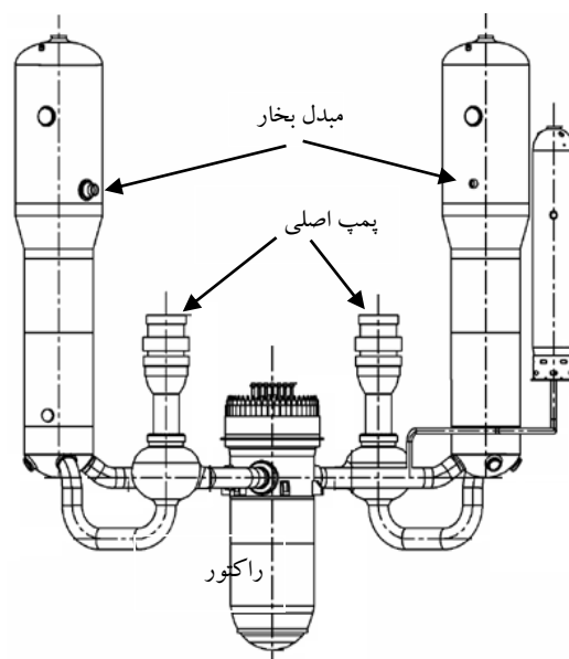
شکل ۱. نمایی از مدار اولیه‌ی نیروگاه هسته‌ای IR-360 و نحوه‌ی ارتباط اجزای اصلی آن [۲۱].
