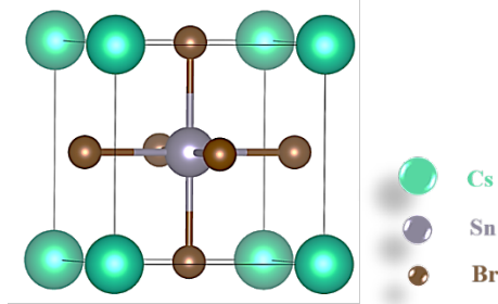
شکل ۲. ساختار کریستالی CsSnBr 3 .
