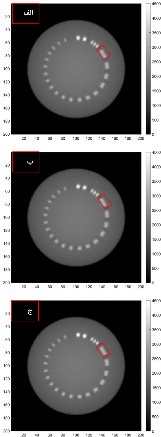
شکل ۱۳. تصویر حاصل از بازسازی پروجکشن‌های انتگرال نهشت انرژی با اعمال تخمین‌گرهای مسیر الف (SLP، ب) CSP و ج) MLP در ابعاد پیکسل ۱ میلی‌متر.
