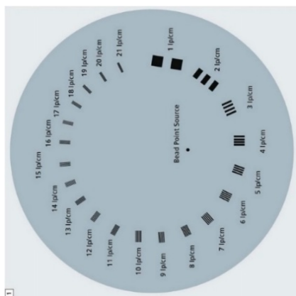
شکل ۲. فانتوم استاندارد حد تفکیک بالای Catphan \delta 28 [۲۳].
