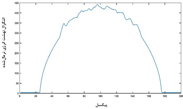
شکل ۱۰. پروفایل پروجکشن انتگرال نهشت انرژی اصلاح شده در زاویه صفر درجه.
