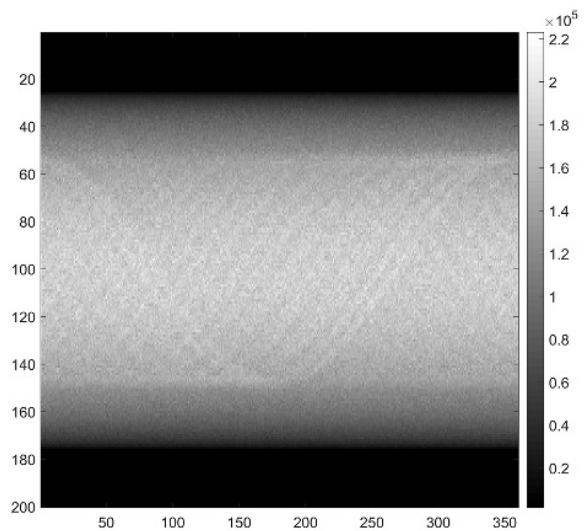
شکل ۸. سینوگرام در الگوریتم FBP.
