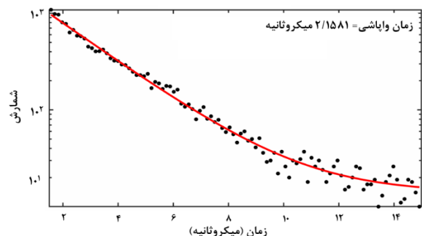
شکل ۱۱. تابع توزیع زمان واپاشی میون حاصل اندازه‌گیری تجربی میون‌های کیهانی به مدت ۲۱ روز با شناسایی ۱۲۲۷۰ تا میون.
