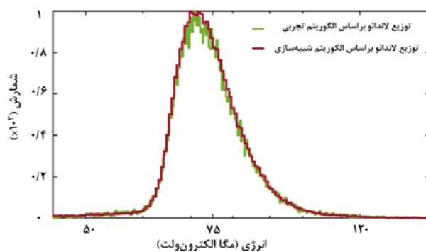
شکل ۸. توزیع لاندائو (انرژی به‌جای‌مانده از میون‌های عبوری) با استفاده از هر دو الگوریتم پردازش شبیه‌سازی و تجربی به‌ازای ۱۱۱۵۰ رویداد میون.
