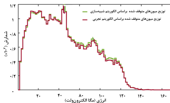
شکل ۹. طیف انرژی میون‌های متوقف‌شده در آشکارساز می‌نی‌ایراند با استفاده از دو الگوریتم پردازش شبیه‌سازی و تجربی به‌ازای ۱۱۱۵۰ رویداد میون.
