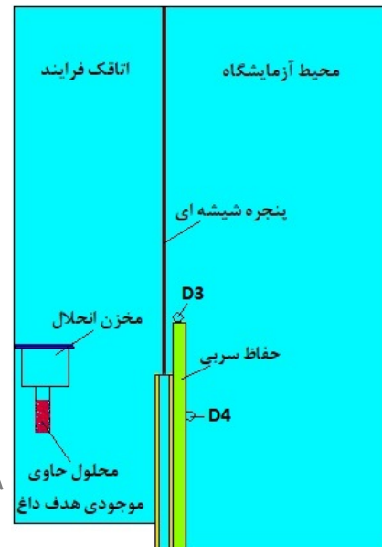
شکل ۴: اتاقک فرایند شبیه‌سازی شده توسط کد MCNPX
