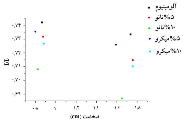
شکل ۵. عبور نسبی تابش نوترون برحسب ضخامت حفاظ Al-B_4C
