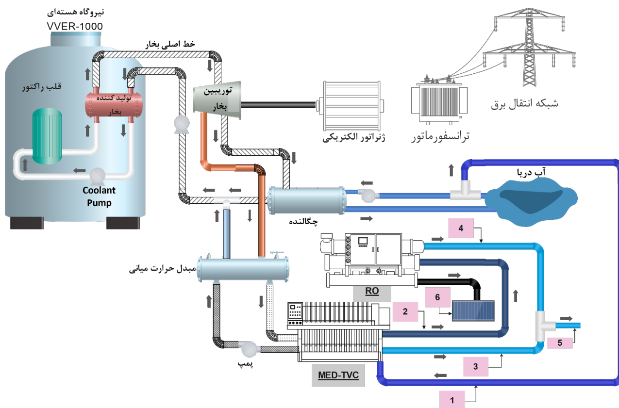
شکل ۱. شماتیک کوپلینگ سیستم هیبرید آب شیرین کنی و نیروگاه هسته‌ای.
