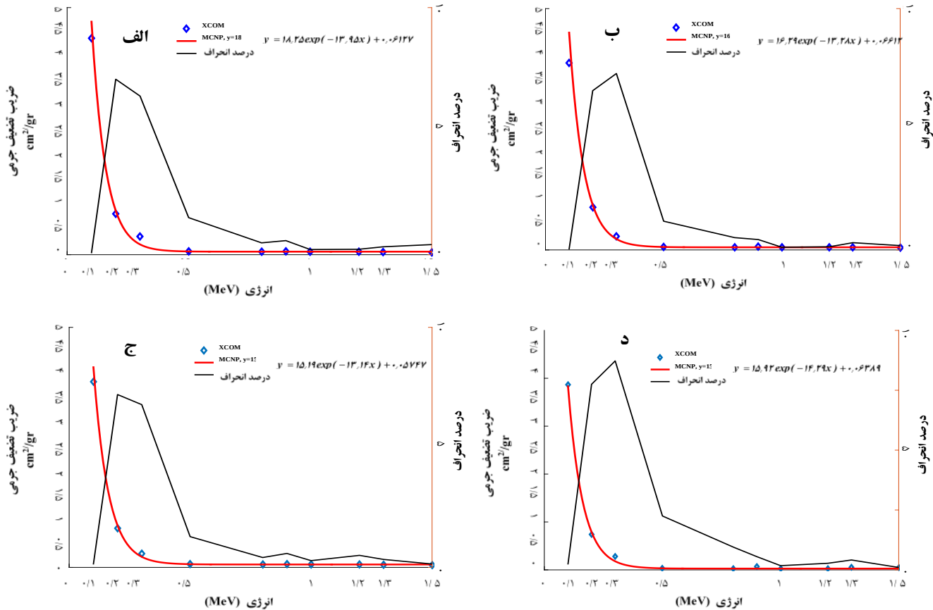
شکل ۳. تغییرات \mu_m نمونه شیشه بر حسب انرژی اشعه گاما برای (الف) C ۱ ، (ب) C ۲ ، (ج) C ۳ و (د) C ۴ .
