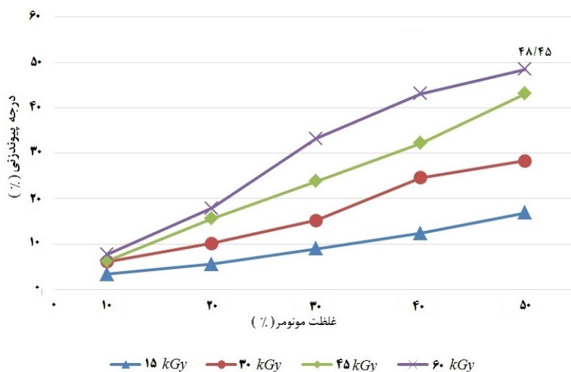
شکل ۹. تغییرات درصدهای پیوندزنی با روش هم‌زمانی در حضور نمک فریک کلراید ۰/۱۵٪ در غلظت‌های مختلف مونومر عاملی.
