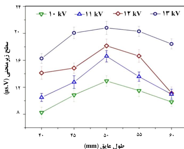
شکل ۷: شدت باریکه‌ی یون در طول‌های مختلف عایق از جنس پیرکس با هندسه‌ی آند مخروطی و در ولتاژهای مختلف تخلیه‌ی الکتریکی ۱۰ تا ۱۳ kV و فشار ۴mbar.
