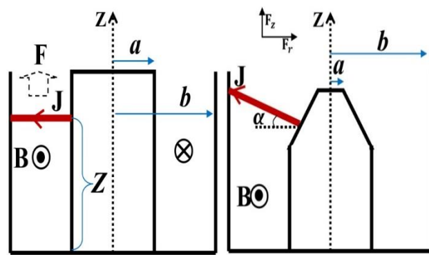
شکل ۹. مؤلفه‌های نیروی لورنتس برای دو آند مخروطی و استوانه‌ای.
