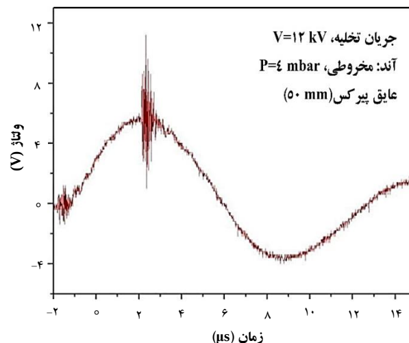
شکل ۴. سیگنال جریان تخلیه‌ی الکتریکی حاصل از پیچ‌های روگوفسکی برای آند مخروطی - عایق پیرکس در ولتاژ ۱۲kV و فشار ۴mbar.
