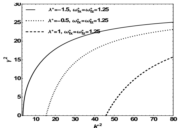
شکل ۲. مربع آهنگ رشد ناپایداری رایلی-تیلور برحسب مربع عدد موج به ازای پارامترهای ثابت مشترک ( \omega_{fx}^* = \omega_{fz}^* = 1.25 ) و پارامتر ثابت آزاد \lambda^* = -1.5, -0.5, 1
