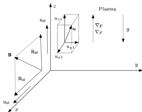
شکل ۱. ارتباط بین مقادیر مختلف مربوط به ناپایداری رایلی-تیلور؛ کمیت‌های \vec{B} ، \vec{u} ، \vec{g} و \nabla p به ترتیب میدان مغناطیسی، سرعت جریان تعادلی، شتاب گرانش، گرادیان فشار و گرادیان چگالی هستند.
