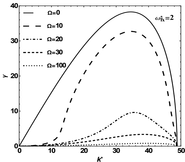
شکل ۳. آهنگ رشد ناپایداری رایلی-تیلور برحسب عدد موج به ازای پارامتر ثابت مشترک \omega_{fx}^* = 2 و پارامتر ثابت آزاد (\Omega = 0, 10, 20, 30, 100) .
