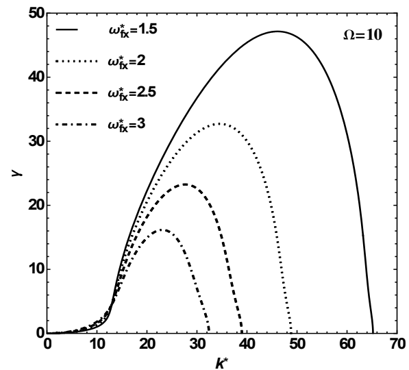
شکل ۴. آهنگ رشد ناپایداری رایلی-تیلور بر حسب عدد موج به ازای پارامتر ثابت مشترک \Omega=10 و پارامتر ثابت آزاد (\omega_{*x}=1.5, 2, 2.5, 3) .
