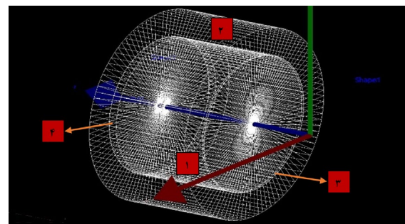
شکل ۳. هندسه‌ی مجموعه‌ی آشکارساز شبیه‌سازی شده؛ (۱) قسمت ماده‌ی سوسونز؛ (۲) محفظه‌ی پوشش‌دهنده‌ی مجموعه‌ی آشکارساز؛ (۳) پنجره‌ی جلویی و (۴) پنجره‌ی پشت آشکارساز.
