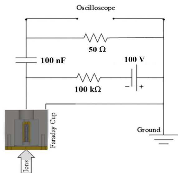
شکل ۱. مدار راه انداز فارادی کاپ که این آشکارساز را در ولتاژ ۱۰۰V به صورت معکوس بایاس می کند.
