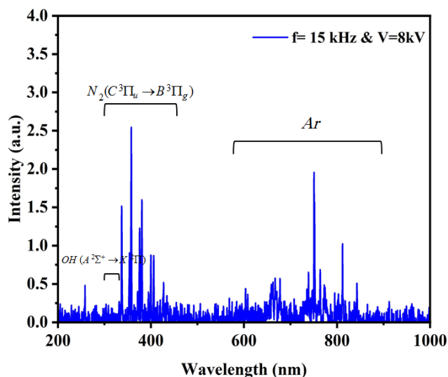
شکل ۲. طیف انتشار نوری را در محدوده ۲۰۰ تا ۱۰۰۰ nm.
