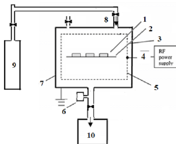
شکل ۱. دستگاه پلاسمایی مورد استفاده و شماتیک آن، (۱) نمونه چیده شده، (۲) سینی‌های نگه‌دارنده، (۳) منطقه پلاسما، (۴) شبکه تطبیق، (۵) الکتروود شبکه‌ای، (۶) فشارسنج، (۷) الکتروود (چمبر)، (۸) پورت هوادهی، (۹) سیستم تزریق گاز (شامل کپسول گاز، لوله‌های ارتباطی و شیرهای سوزنی)، (۱۰) پمپ خلأ.
