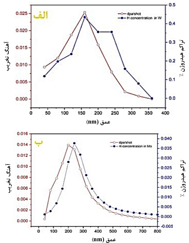
شکل ۶. الف) نمودار کمی آسیب تابش برحسب شات و تراکم هیدروژن برحسب عمق تنگستن، ب) نمودار کمی آسیب تابش برحسب شات و تراکم هیدروژن برحسب عمق مولیبدن.
