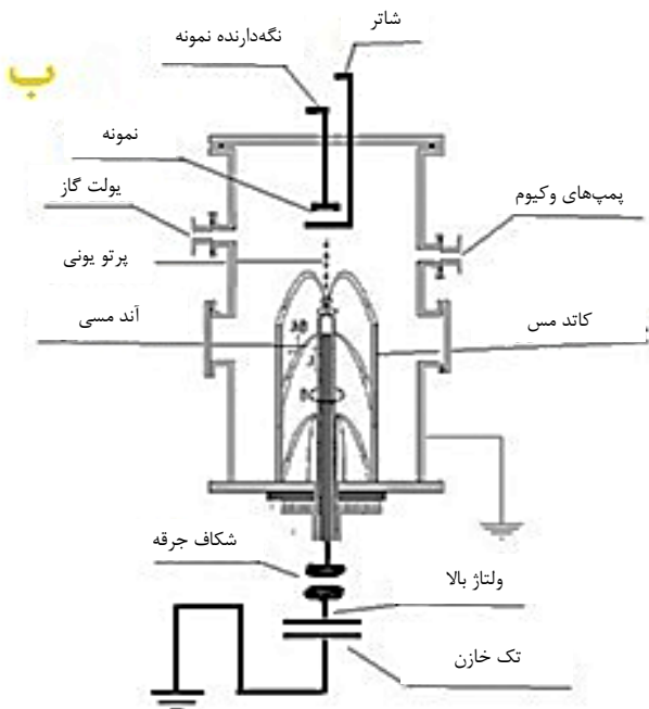
شکل ۱. الف) طرح‌واره دستگاه پلاسمای کانونی MTPF-۲، ب) آرایه آند و کاتدهای دستگاه پلاسمای کانونی.
