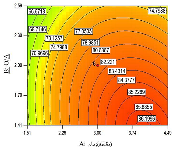
شکل ۱۰. تأثیر پارامترهای نسبت فاز آلی به آبی و زمان اختلاط در تهی‌سازی.
