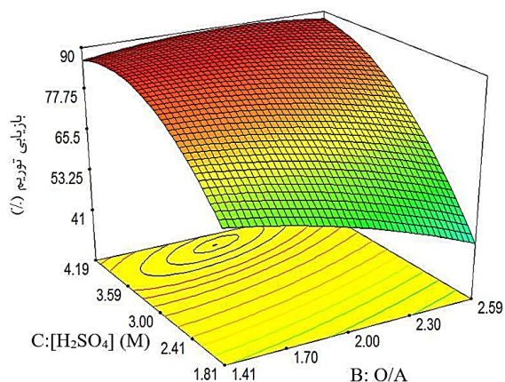
شکل ۱۳. میزان تهی‌سازی توریم در نقاط بهینه.
