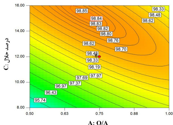
شکل ۳. تأثیر نسبت فاز آلی به آبی و درصد حلال در فرایند استخراج حلالی.
