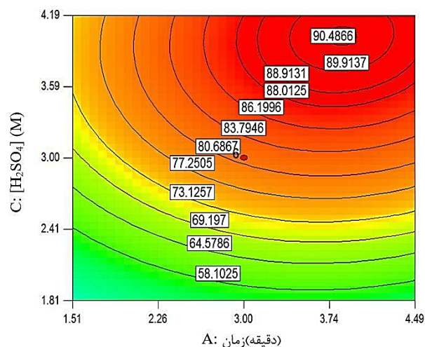
شکل ۱۱. تأثیر پارامتر زمان اختلاط دو فاز و غلظت اسید سولفوریک در فرایند تهی‌سازی.
