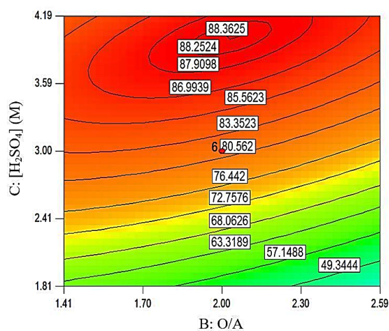
شکل ۱۲. تأثیر پارامترهای نسبت فاز آلی به آبی و غلظت سولفوریک اسید.
