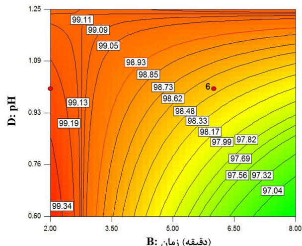
شکل ۹. تأثیر پارامترهای زمان اختلاط و pH محلول لیچ لیکور.
