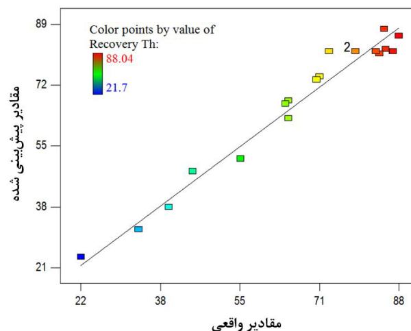
شکل ۹. مقادیر پیش‌بینی شده توسط مدل برحسب مقادیر واقعی در تهی‌سازی توریم.
