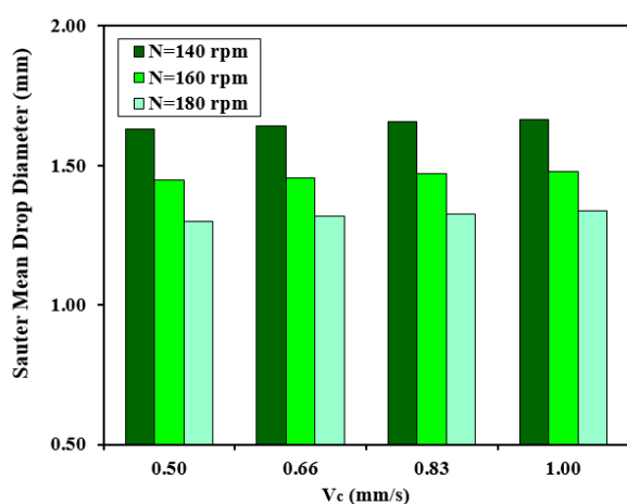
شکل ۴. اثر سرعت فاز پیوسته بر قطر ستر قطره در سیستم استخراج توریم از محلول آبی (سرعت فاز پراکنده برابر با ۰/۶۶ mm/s).
