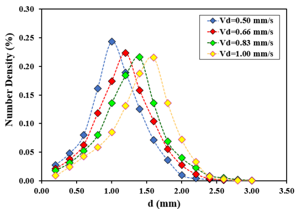
شکل ۶. تأثیر سرعت فاز پراکنده بر روی توزیع اندازه قطرات در سیستم استخراج توریم از محلول آبی (سرعت فاز پیوسته برابر با ۰/۶۶ mm/s و N=160 rpm).
