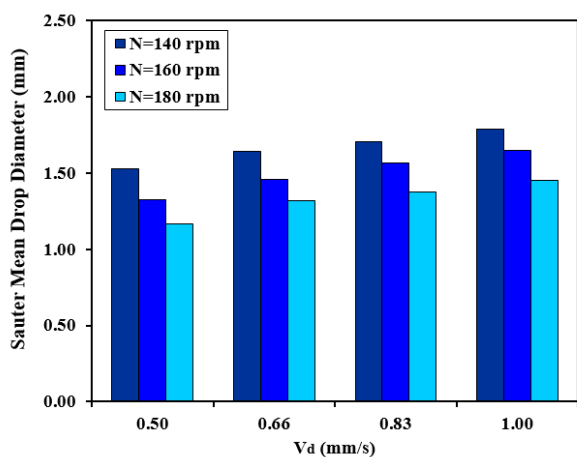
شکل ۳. اثر سرعت فاز پراکنده بر قطر ستر قطره در سیستم استخراج توریم از محلول آبی (سرعت فاز پیوسته برابر با ۰/۶۶ mm/s).
