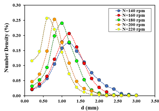
شکل ۵. تأثیر سرعت اختلاط روی توزیع اندازه قطرات در سیستم استخراج توریم از محلول آبی (سرعت فازهای پراکنده و پیوسته برابر با ۰/۶۶ mm/s).
