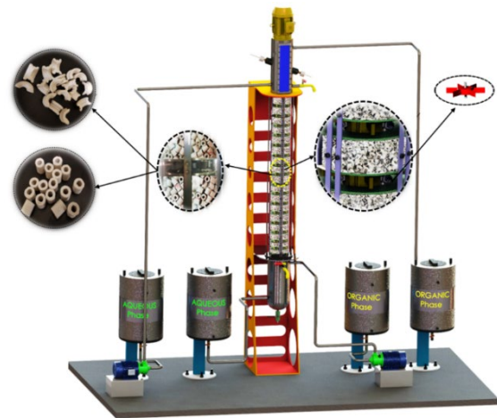
شکل ۱. طرح‌واره از ستون پر شده همزن‌دار به همراه اجزاء جانبی آن.
