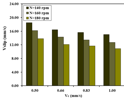
شکل ۱۲. اثر سرعت فاز پیوسته بر سرعت لغزشی برای سیستم استخراج توریم از محلول آبی (سرعت فاز پراکنده برابر با ۰/۶۶ mm/s).
