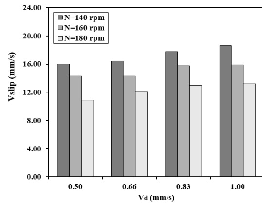
شکل ۱۳. اثر سرعت فاز پراکنده بر سرعت لغزشی در سیستم استخراج توریم از محلول آبی (سرعت فاز پیوسته برابر با ۰/۶۶ mm/s).
