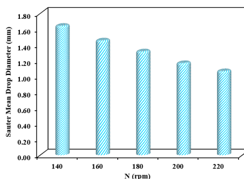
شکل ۲. اثر سرعت اختلاط بر قطر میانگین ستر قطره در سیستم استخراج توریم از محلول آبی (سرعت فازهای پراکنده و پیوسته برابر با ۰/۶۶ mm/s).
