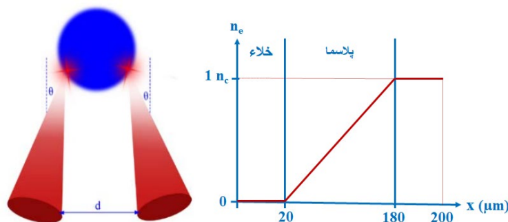
شکل ۱. شماتیک برهم‌کنش دو باریکه لیزری با زوایا و فواصل مختلف که پس از طی ۲۰ میکرون در خلأ با رمپ چگالی وارد پلاسما می‌شوند.
