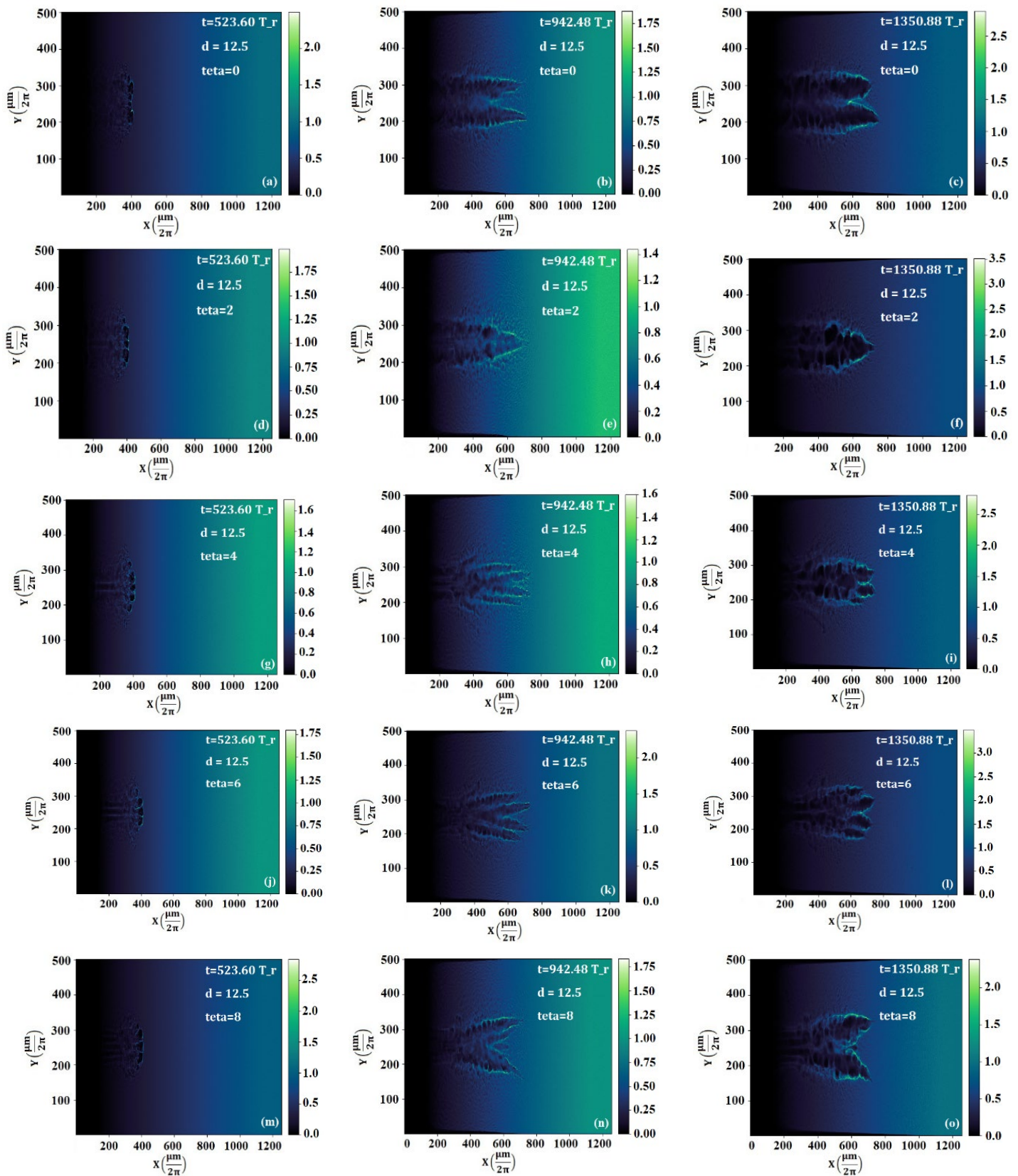
شکل ۵. تحول فضایی- زمانی چگالی پلازما در زمان‌های مختلف به ازای زوایای مختلف.
