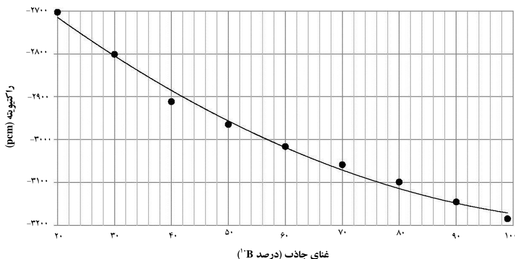
شکل ۱۰. اثر غنی‌سازی بر عملکرد سیستم خاموشی دوم.
