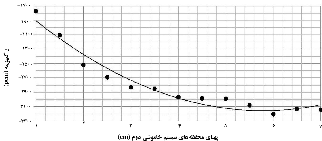
شکل ۸. اثر پهنای سیستم خاموشی دوم حاوی جاذب روی راکتیویته.
