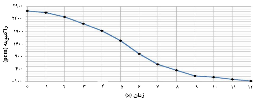
شکل ۴. تغییرات راکتیویته با زمان.
