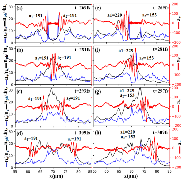
شکل ۴. نمایه میدان عرضی، چگالی عددی الکترون‌ها و فوتون‌ها برحسب مکان در دو حالت (a-d): پالس‌های متقابل با نسبت برابر a_1=a_2=191 و (e-h): نسبت‌های a_1=153 , a_2=229 , a_1=229 , a_2=153 در زمان‌های مختلف.
