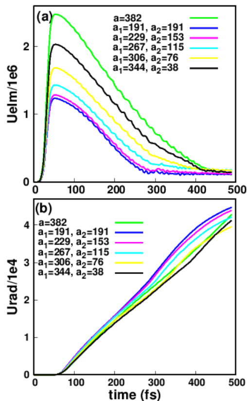
شکل ۹. تغییرات زمانی انرژی الکترومغناطیسی کل به‌نحی که در (a) و (b) نشان داده شده است. (b) تابش شده از سیستم، برای پیکربندی‌های مختلف شرح داده شده در متن.
