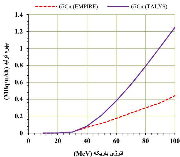
شکل ۱۲. تغییرات بهره تولید ^{67}\text{Cu} با انرژی در واکنش ^{68}\text{Zn}(p, 2p)^{67}\text{Cu} بعد از حذف کامل ^{64}\text{Cu} .
