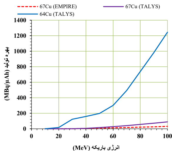
شکل ۱۱. تغییرات بهره تولید ^{67}\text{Cu} و ^{64}\text{Cu} با انرژی در واکنش ^{68}\text{Zn}(p, 2p)^{67}\text{Cu} .
