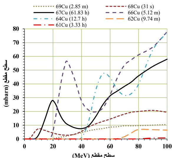
شکل ۷. تابع برانگیختگی رادیوایزوتوپ‌های مس تولید شده در واکنش ^{70}\text{Zn}(d,x)^{67}\text{Cu} حاصل از کد TALYS.
