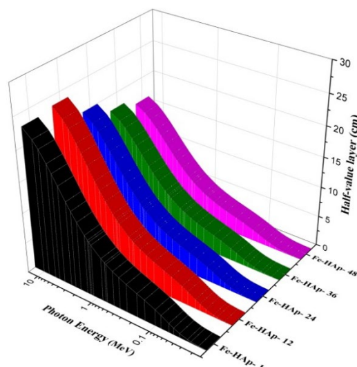
شکل ۷. تغییرات لایه نیم مقدار برای نمونه های منتخب بر حسب تغییرات انرژی.
