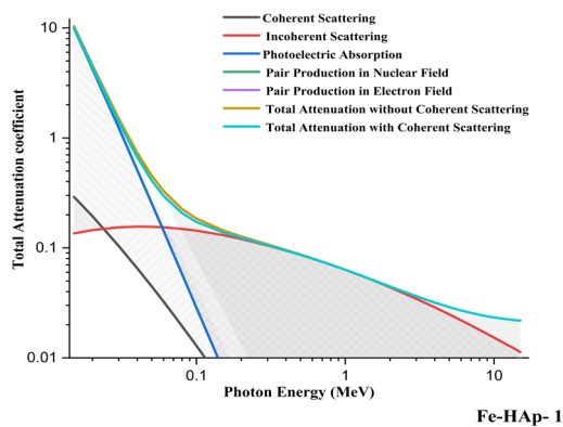
شکل ۲. تغییرات ضریب تضعیف کل برای نمونه Fe-Hap-۱ برحسب تغییرات انرژی.
