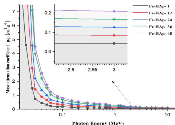
شکل ۳. تغییرات ضریب تضعیف جرمی برای نمونه‌های منتخب برحسب تغییرات انرژی.
