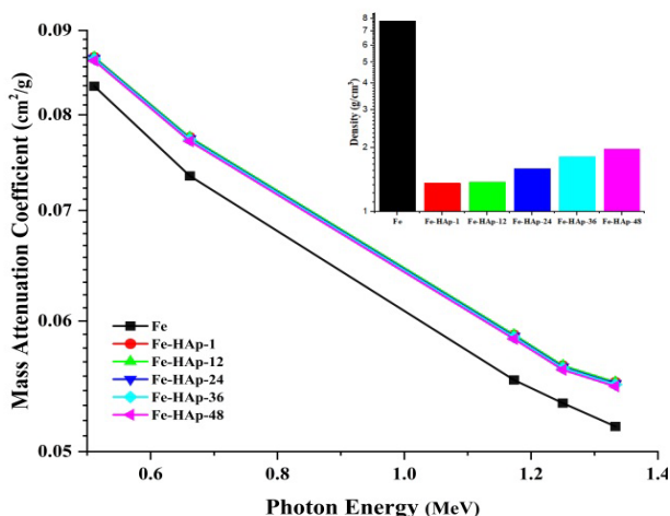
شکل ۴. تغییرات ضریب تضعیف جرمی برای نمونه‌های منتخب با عنصر آهن برحسب تغییرات انرژی.
