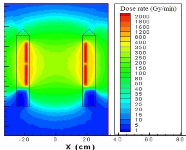
شکل ۵. پروفایل دز داخل هر دو محفظه پرتودهی درونی و بیرونی سامانه پرتودهی پرتابل با ظرفیت ۱۰۰ کیلوگری.
