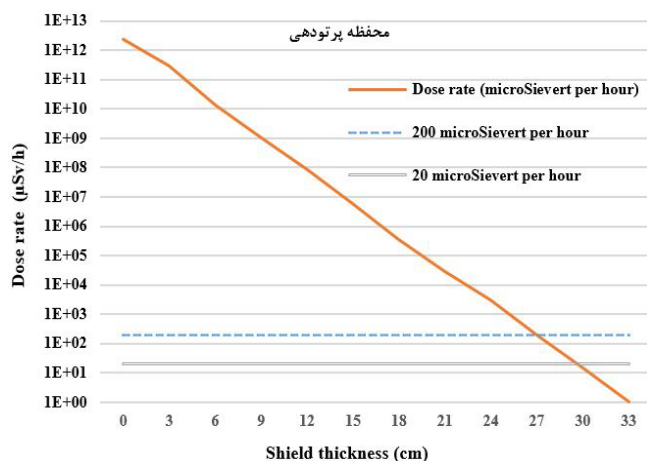
شکل ۶. نمودار آهنگ دز برحسب ضخامت سربی برای محفظه پرتودهی.
