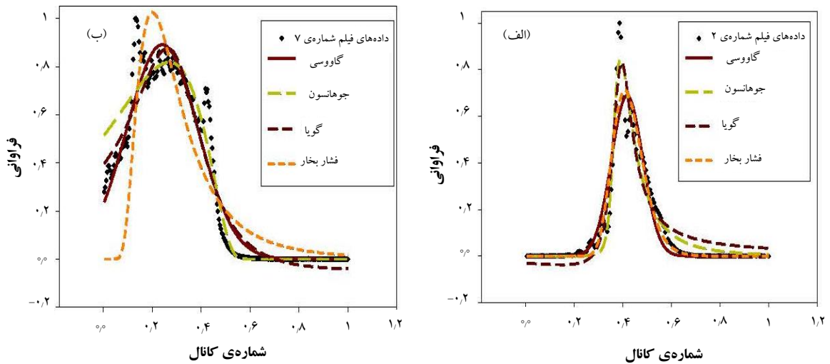
شکل ۵. انطباق منحنی‌های توابع احتمال بر داده‌های مربوط به زمینه فیلم‌های رادیوگرافی.
