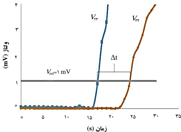
شکل ۶. تغییرات زمانی ولتاژ در مکان‌های مختلف برای اندازه‌گیری V_q به ازای ولتاژ مرجع ۱ mV (شرایط اولیه: E_{pulse}=58.32 J، T_{op}=81 K، I_{op}=55 ).
