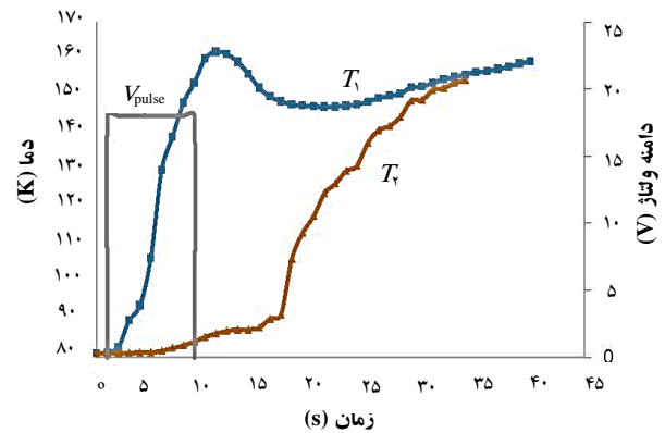
شکل ۸. تغییرات زمانی دمای T_1 و T_2 به ازای انرژی اختلال E=58.32 J.
