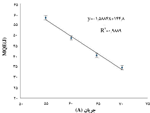
شکل ۷. انرژی فرونشانی برحسب جریان در بازه‌ی ۵۵ تا ۷۰ A در دمای T_{op}=81 K.
