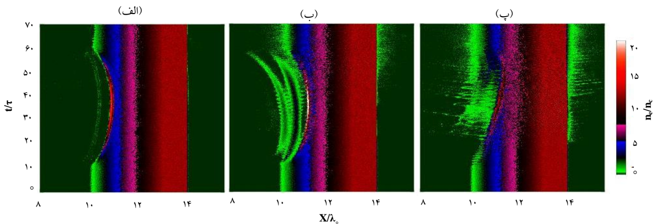
شکل ۶. تحولات زمانی چگالی الکترون‌ها در برهم‌کنش با پالس بدون چِرپ (الف)، چِرپ منفی (ب) و چِرپ مثبت (پ).
