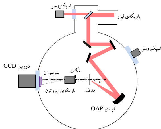
شکل ۱. طرحی از چیدمان آزمایش.
