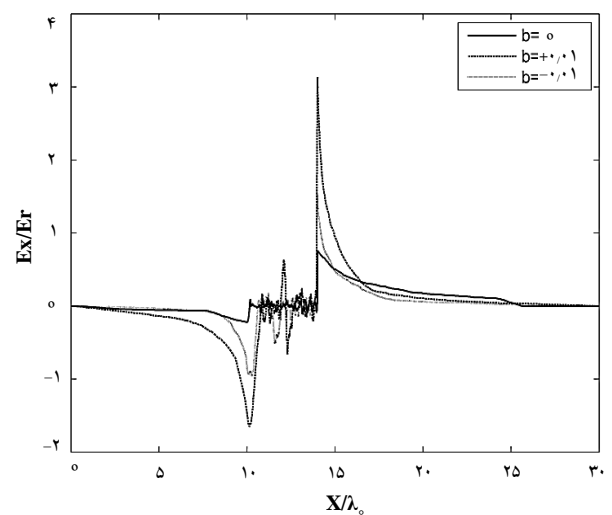
شکل ۷. تغییرات میدان الکترواستاتیکی برای حالت‌های مختلف چِرپ b = 0, +0.01, -0.01 .
