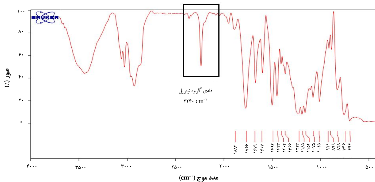
شکل ۳. طیف زیرقرمز الیاف اصلاح شده‌ی پلی استایرن- آکریلونیتریل قبل از تبدیل گروه‌های نیتریل به آمیدوکسیم (شدت قله‌ی متناظر با گروه نیتریل ۵۰٪).
