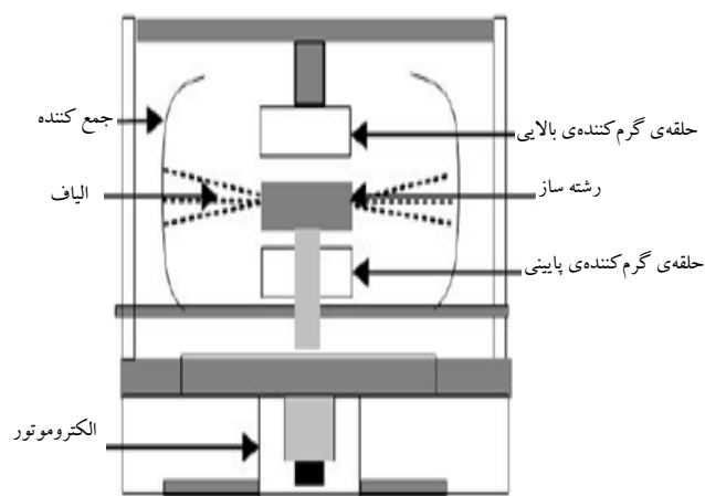
شکل ۱. طرح‌واره‌ی دستگاه نیرویسی.
