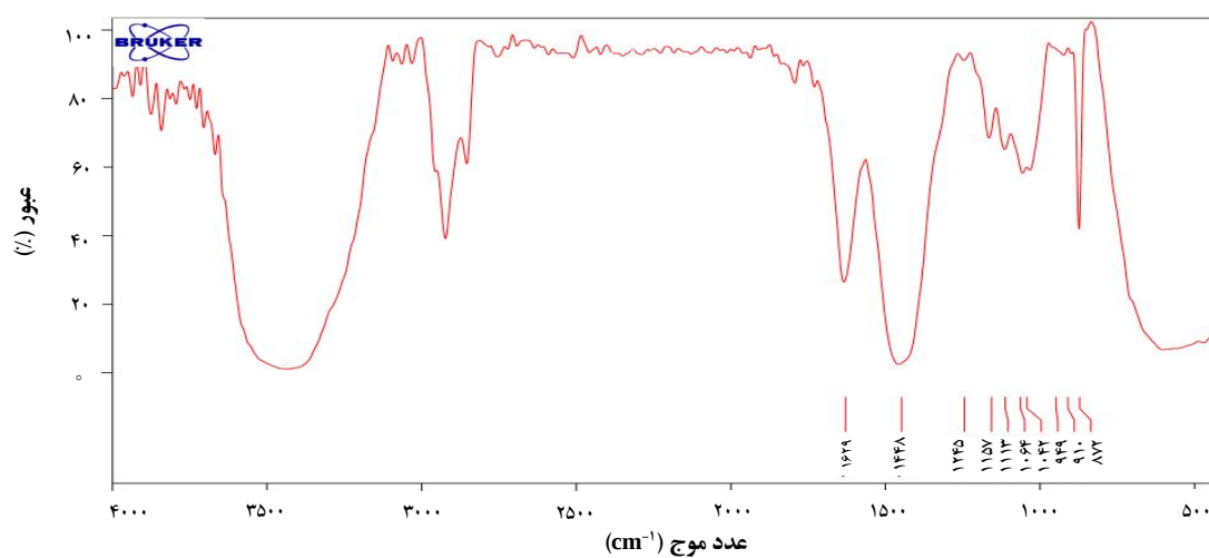
شکل ۵. طیف الیاف اصلاح شده‌ی پلی استایرن- آکریلونیتریل بعد از تبدیل گروه‌های نیتریل به آمیدوکسیم ۷۲ ساعت بعد از شروع فرایند تبدیل گروه (شدت قله‌ی گروه نیتریل ۰٪).
